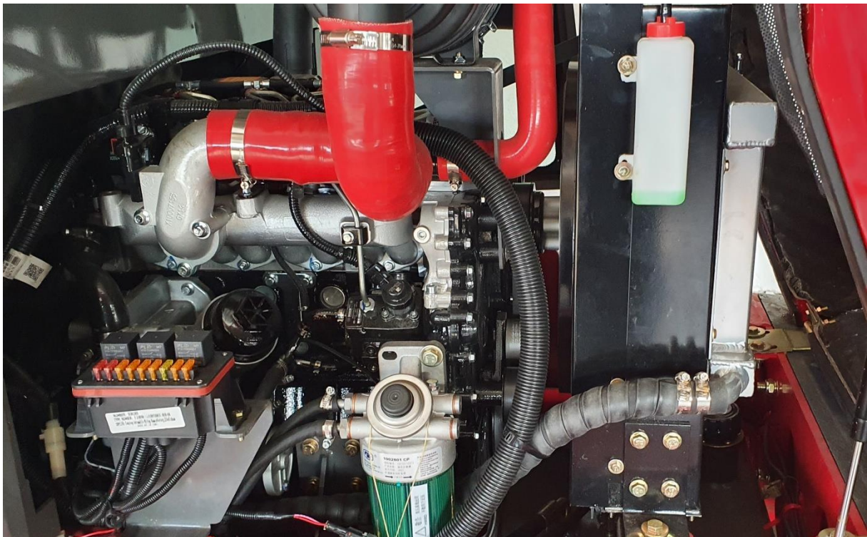
Motor Yunnice: 2 liter 4 cylindrar upp till 50 hk !
